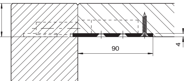
Schnitt A-A Cross-section A-A Coupe A-A Sección A-A
