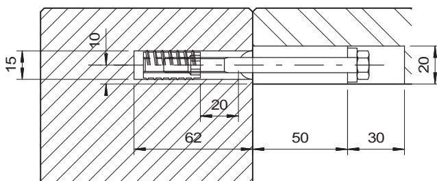
Schnitt B-B Cross-section B-B Coupe B-B Sección B-B
