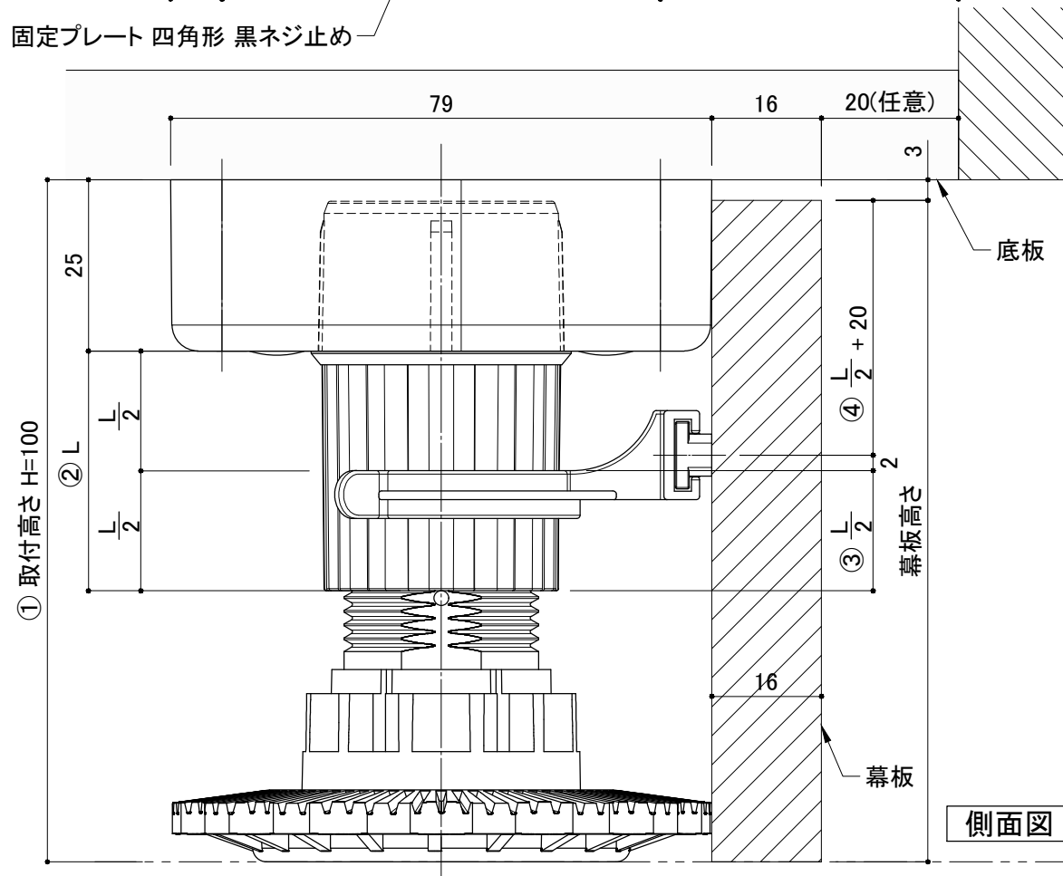
固定プレート四角形ネジ止め/幕板クリップ 1個 納まり図
